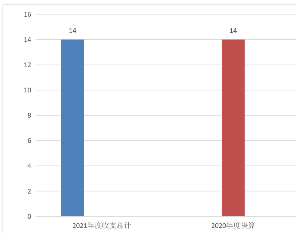
图 1: 收入支出决算对比图
